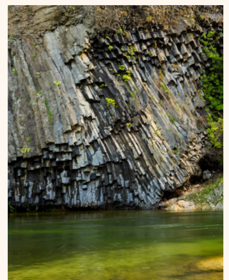
Coulées basaltiques
